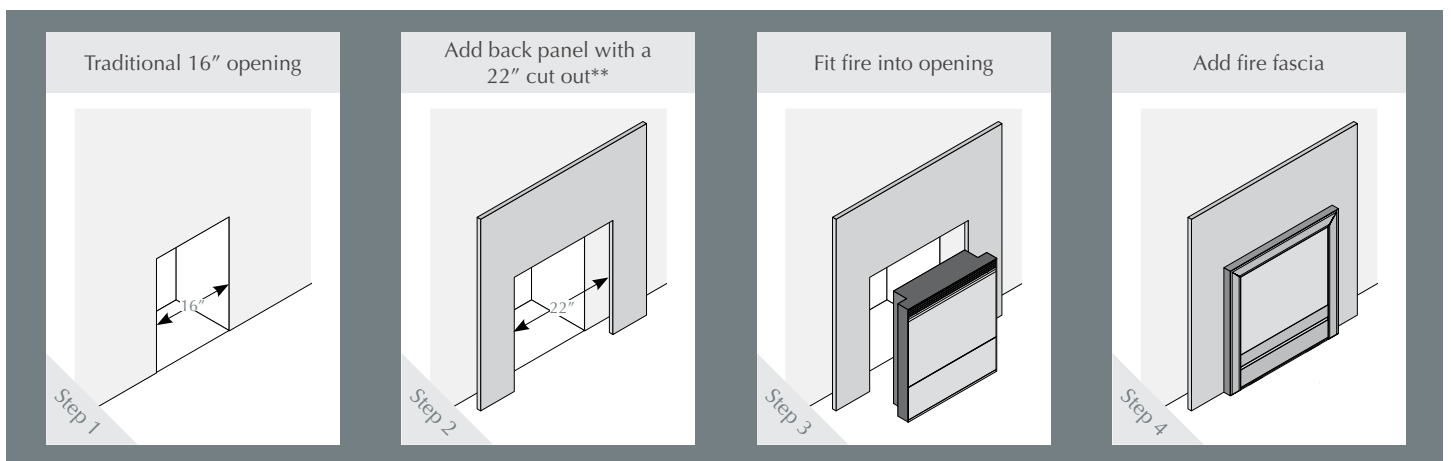
Edge Chrome
